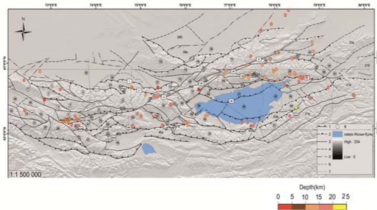
Рисунок 1 – Карта-схема новейших блоков Северного Тянь-Шаня.
