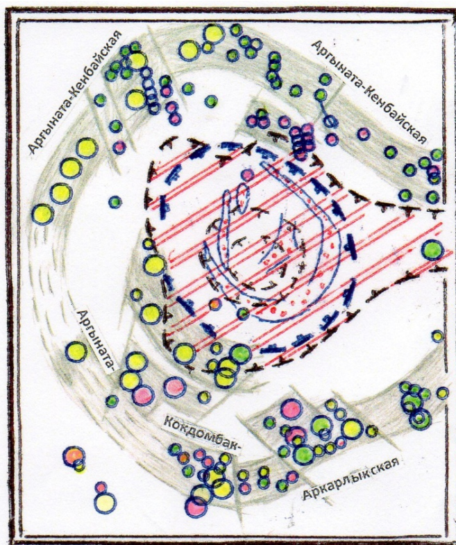
Рисунок 6 – Предполагаемые минерагенические зоны в области влияния Аргынатинского интрузивного массива. Условные обозначения см. рисунок 7
