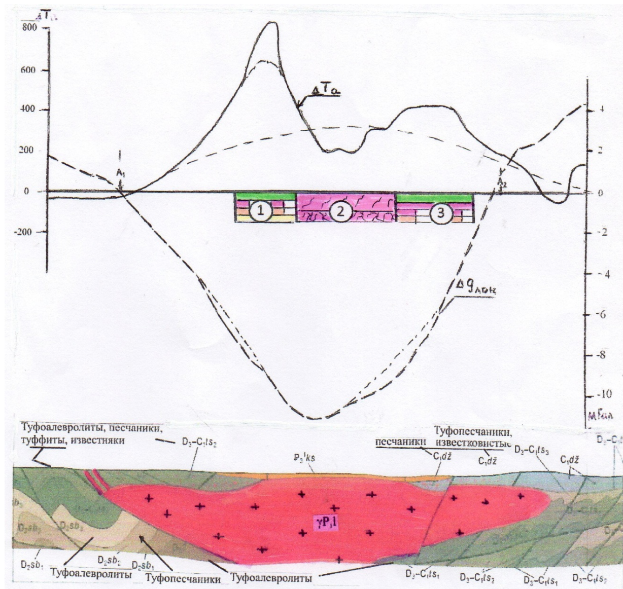
Рисунок 5 – Геолого-геофизический разрез через Аргынатинский интрузивный массив (по Уваровой, Бектасову, Акылбекову): 1–3 – область прогнозирования: 1 – медно-молибденового, скарново-вольфрамового и скарново-магнетитового оруденения с сопутствующим висмутом и оловом, 3 – медно-молибденового, редкометалльного, скарново-вольфрамового и скарново-магнетитового оруденения
