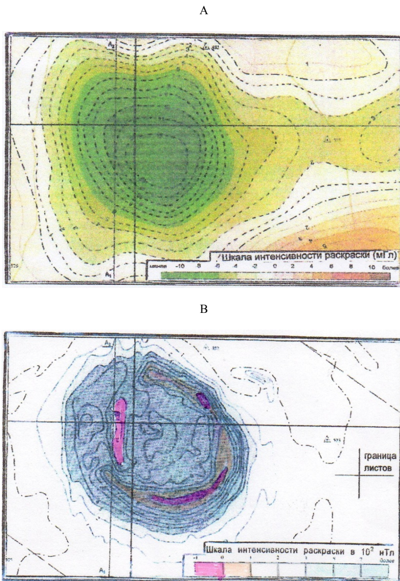
Рисунок 4 – Карта остаточных аномалий силы тяжести при R_{gsz} = 18 км (А), карта аномального магнитного поля \Delta T_a (Б) района Аргынтинского интрузивного массива (по Бектасову, по карте масштаба 1:200 000)
