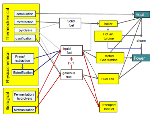
Рисунок 3 – Различные пути для превращения биогаза в энергию
