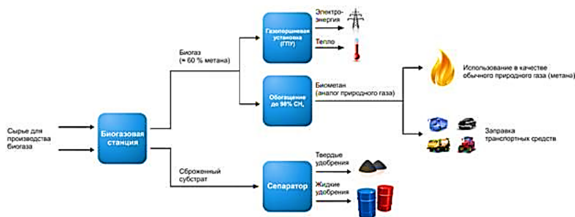
Рисунок 2 – Система получения и сжигания биогаза
