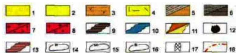
Рисунок 1 – Геологическая карта месторождения Катпар (Губайдулин Ф.Г., 2004)
