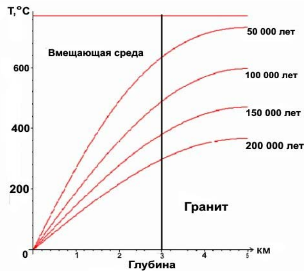
А – температурное поле гранитного массива прогрессивного (дорудного) этапа; Б – температурное поле гранитного массива регрессивного (рудного) этапа; В – пространственное распределение температуры на месторождении Катпар и время становления рудоносной интрузии и процесса рудообразования.
