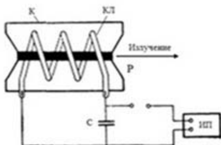
Рисунок 17 – Схема рубинового лазера:
